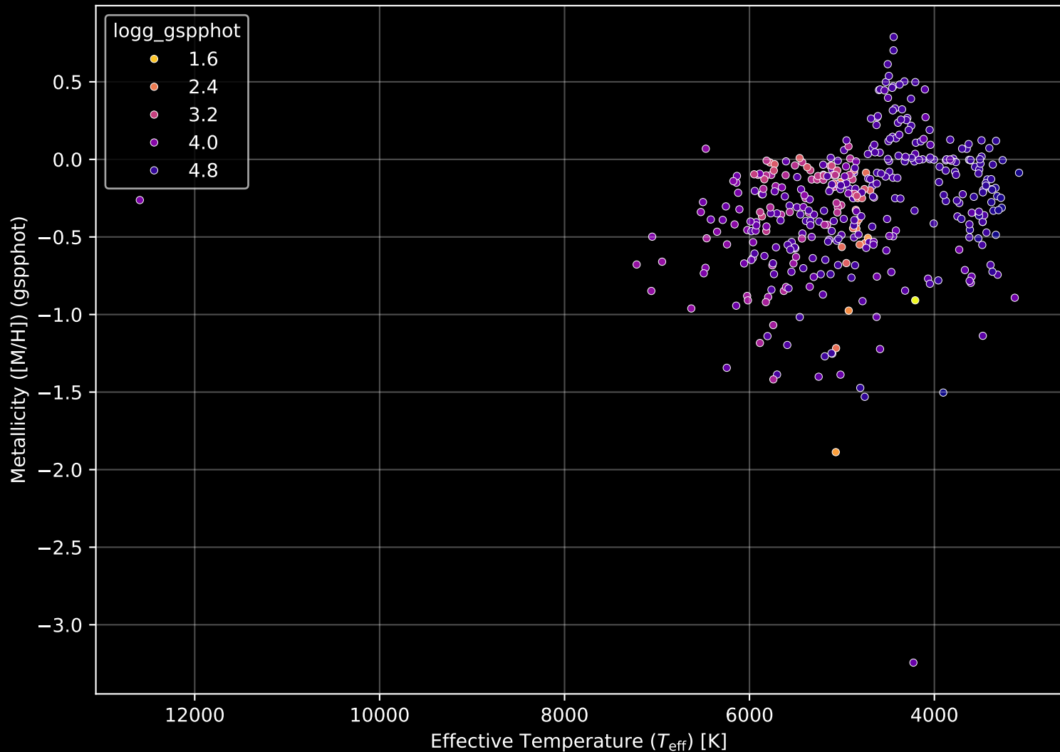
APOGEE DR17 Field: [240+75] Stellar Population Parameters (n= 402)
